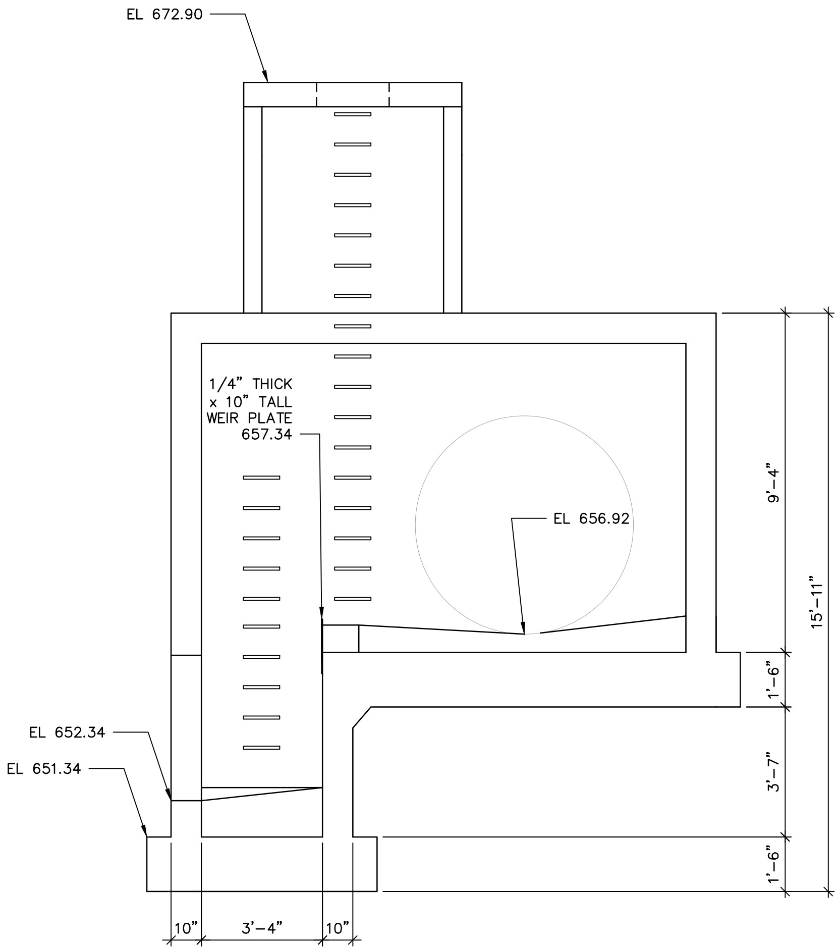
1 SECTION SCALE: 3/8" = 1'-0"
